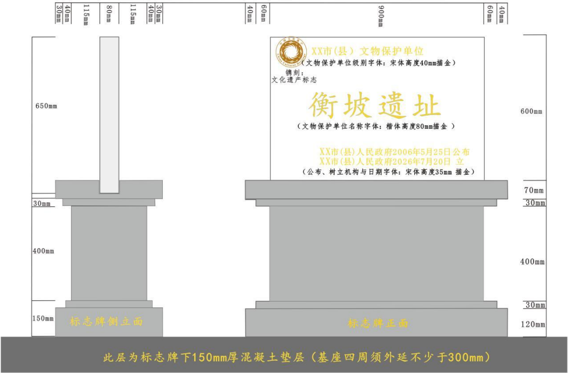
标志牌正、侧面样式尺寸效果图
