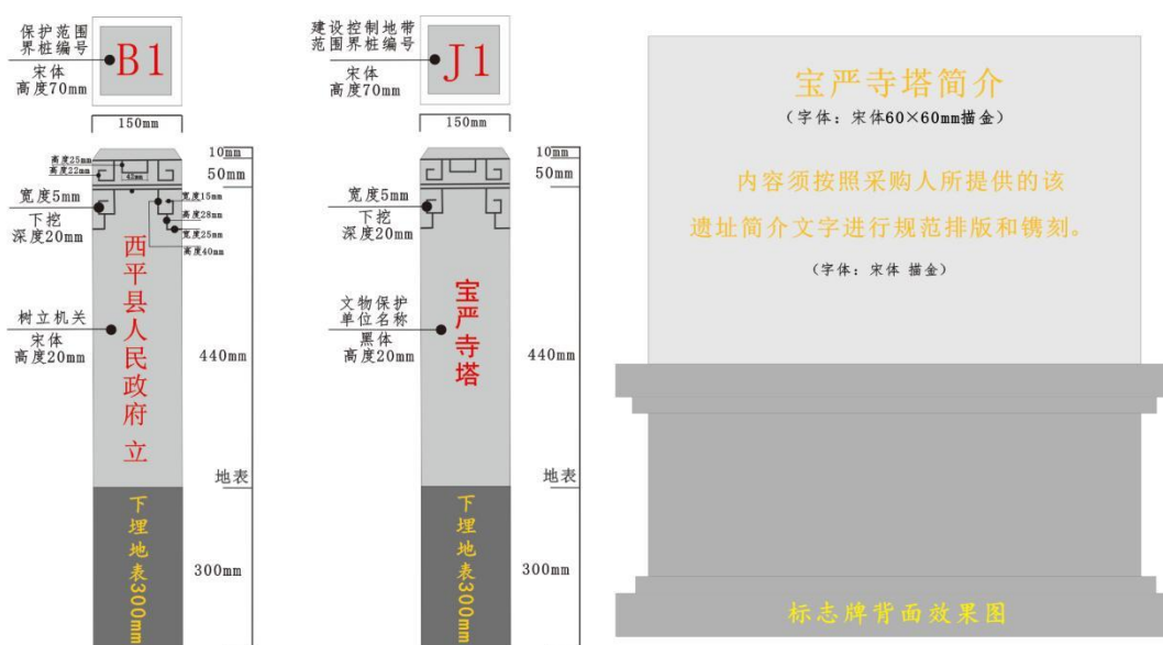
标志牌背面样式尺寸效果图
