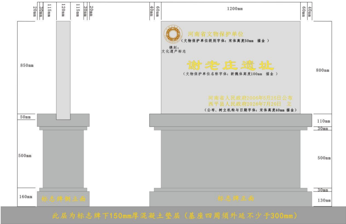
标志牌正、侧面样式尺寸效果图
