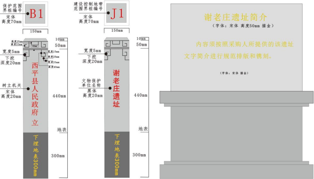
界桩样式尺寸效果图
