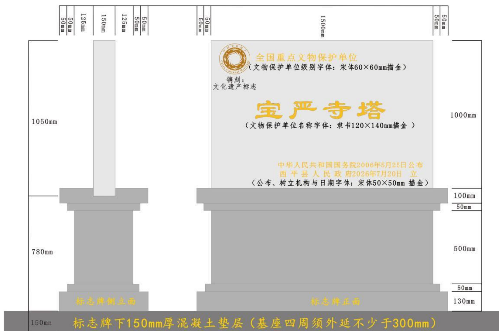
标志牌正、侧面样式尺寸效果图
