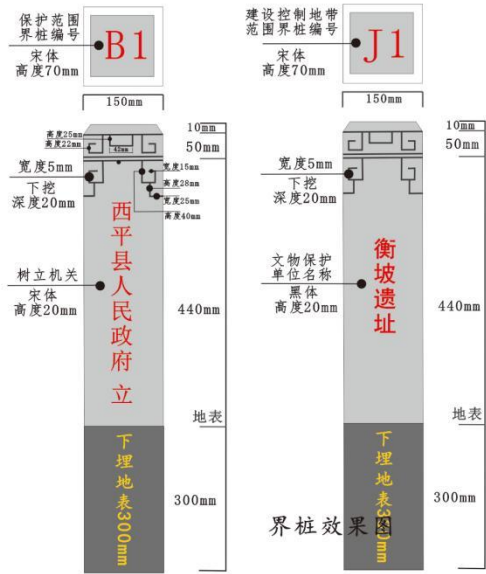
界桩样式尺寸效果图
